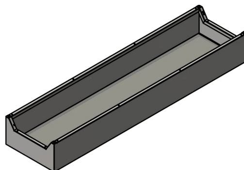
Strøkkasse Galvanisert L600 x H300 x D2400 mm Art. nr.: 595123
